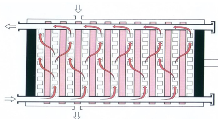
Passage du liquide dans un filtre à plaques
